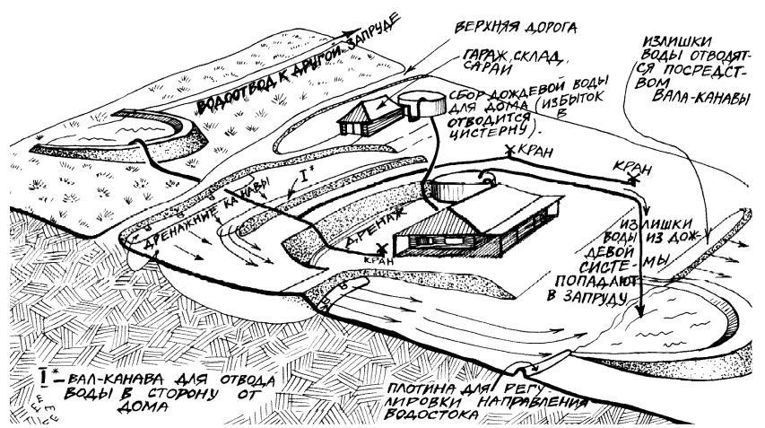
Рис. 2. Идеальный пример взаиморасположения систем водоснабжения, строений и дорог. Валы-канавы служат для отвода воды по горизонталям склона, что способствует уменьшению степени эрозии во время выпадения обильных осадков.
