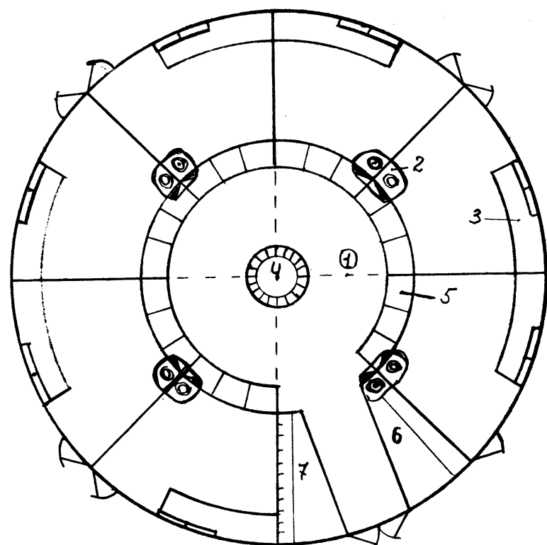
Диаметр внешний — 12 м, диаметр внутренний — 6 м. Высота первого этажа — 3–4 м, второго — 3–3,5 м.
